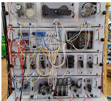
Modell Einspritzanlage
